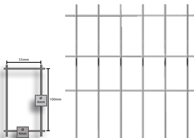
Maille du panneau Zéphyr®
