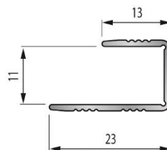
Modèle 10 / 11 mm
