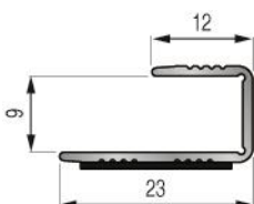
Modèle 8 / 9 mm
