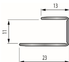
Modèle 10 / 11 mm
