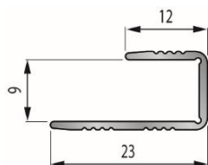
Modèle 8 / 9 mm
