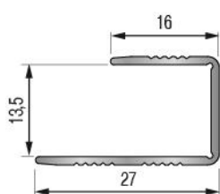
Modèle 12,5 / 13,5 mm
