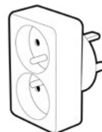
ADAPTATEUR ENTREE 2X2P+T 16A SORTIE 2P+T 20A 4400W BLANC
