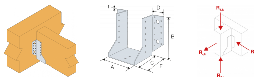
Valeurs Caracteristiques - Bois sur bois - Clouage partiel
