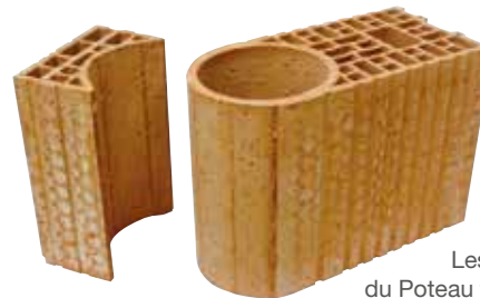
Séparation des 2 éléments du Poteau tableau multi-angles.
