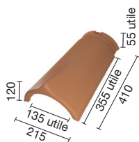
E000 0900 Faîtière-arêtier galbé (2,8 au ml)
