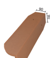
EPE18 7040 Demi-tuile à rabat G + D ❶ (3,3 au ml)
