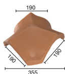
E000 5352 Rencontre 3D femelle
