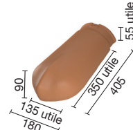
E000 0960 About arêtier galbé
