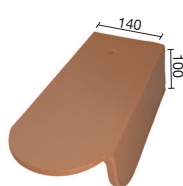
EPE18 7090 Tuile à rabat D (3,3 au ml)
