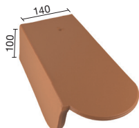
EPE18 7080 Tuile à rabat G (3,3 au ml)
