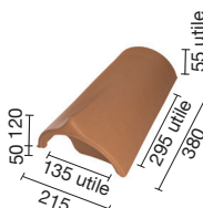
E000 0910 About faîtière galbée début
