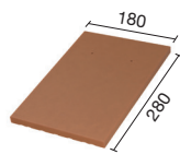
EPE18 8300 Tuile d'égout (5,5 au ml)
