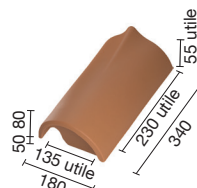
E000 0920 About faîtière galbée fin
