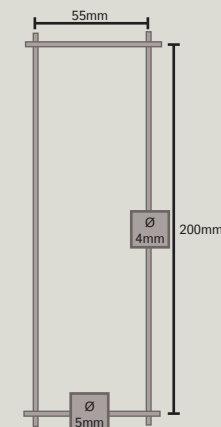
Maille du panneau AQUILON® 45 Medium
