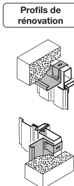
Traverse supérieure
