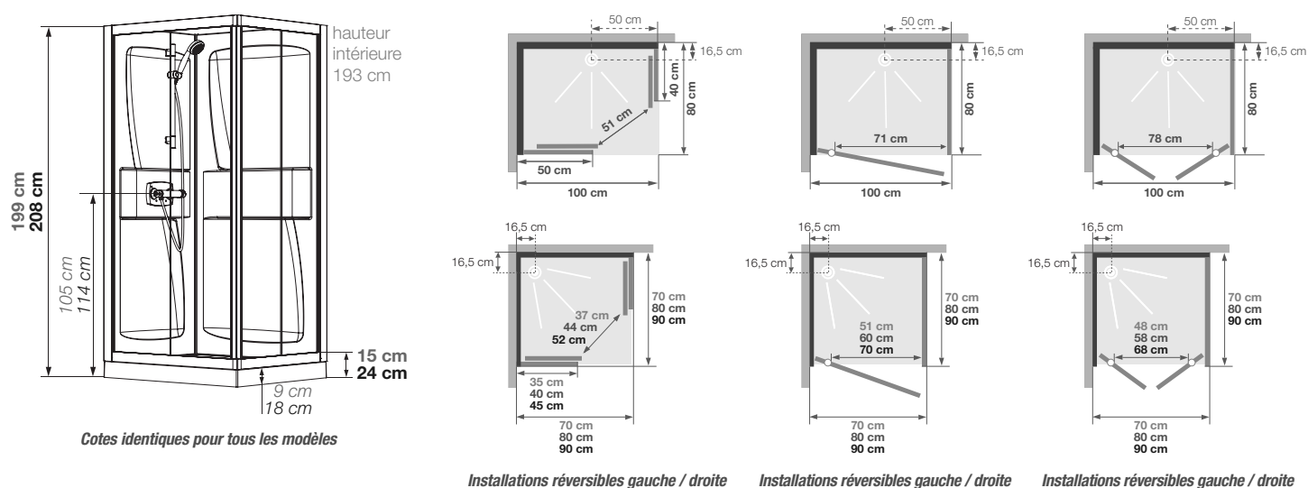
Kineprime 100 x 80 angle - version thermostatique - portes coulissantes
