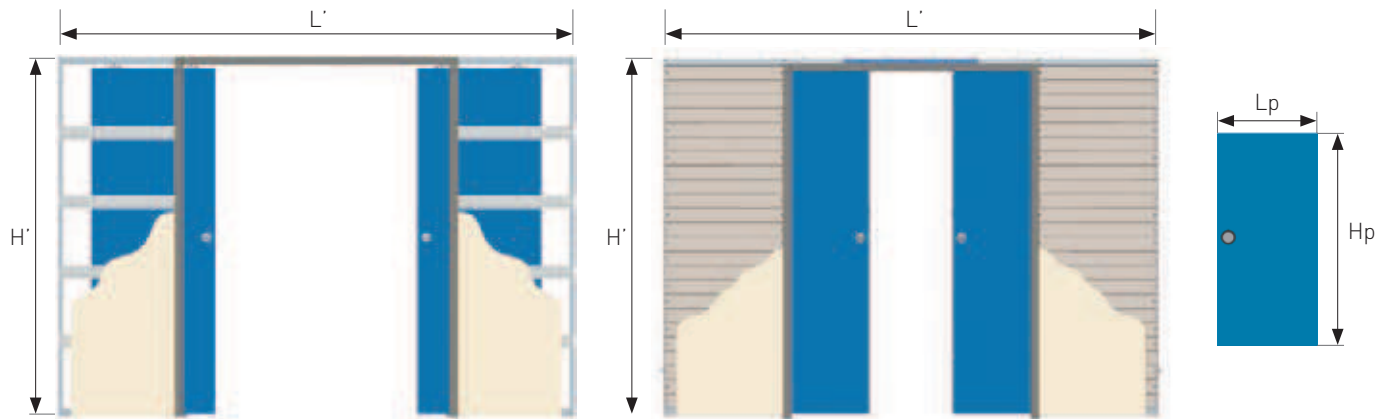
Châssis pour porte à chant droit de 40 mm d'épaisseur (maxi).
