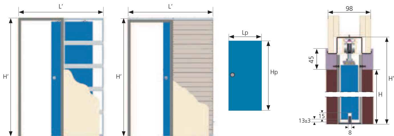
Châssis pour porte à chant droit de 40 mm d'épaisseur (maxi).
