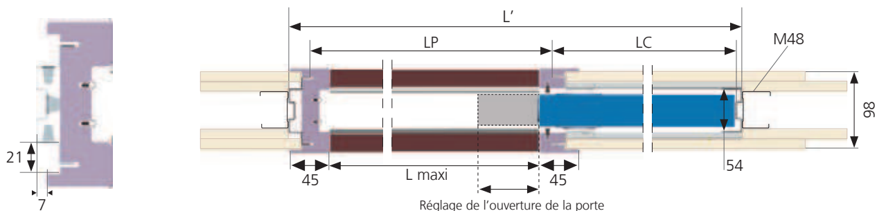
Réglage de l'ouverture de la porte
