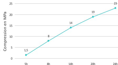
Montée en résistance de la chape à la compression
