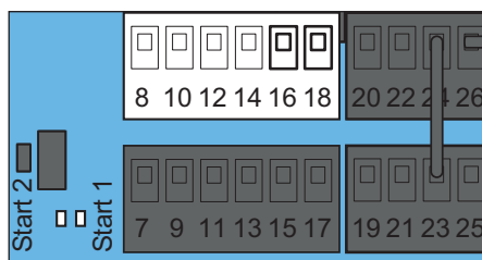
III. Raccords d'un relais multifonction
