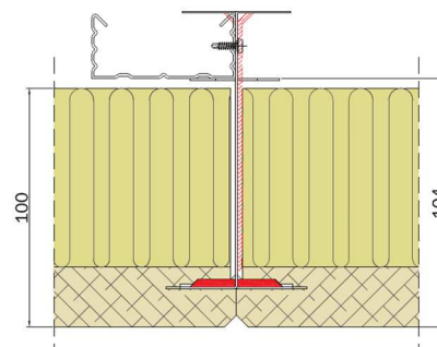
Exemple de fixation sur ossature CD60 avec Clip FMIV INT 125-100/CD60 (2)
