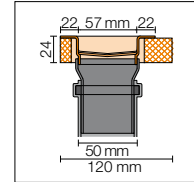
Coupe transversale – Montage le long d'un mur
