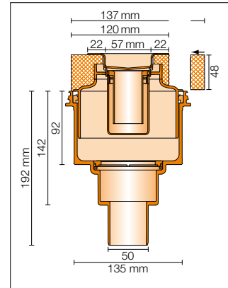
Coupe transversale
