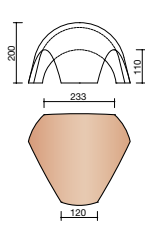
M000 5320 * Rencontre base poignon 3 directions
