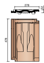
MOPT 8640 Tuile chatière (36 cm 2 ) (0,07 pc / m 2 projeté) ❖
