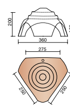
B000 5335 * Rencontre base poignon ÉLEGANTE 3 directions faîtières demi-rondes
