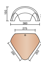
B000 5330 * Rencontre base poignon 3 directions faîtières demi-rondes
