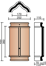
M000 1330 Faîtière double emboîtement standard
