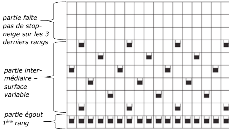
2 stops-neige/m 2
