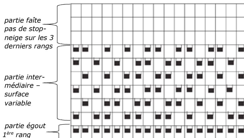
6 stops-neige/m 2
