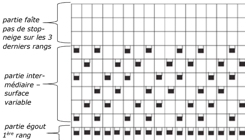
4 stops-neige/m 2
