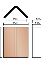
A000 1800 * Faîtière angulaire 90° (3,0 au ml)
