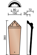
A000 3810 * About d'arêtier de chevauchement "tige de botte"
