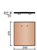
AAR7 8020 Tuile et demie 24 x 27 (5,0 au ml)
