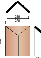
A000 1810 * About de faîtière angulaire
