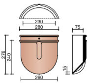
P000 1260 About arêtier 1/2 rond 230 mm
