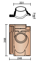
P401 8740 Tuile à douille Ø 100 mm (extraction 78 cm 2 )
