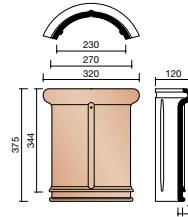
P000 1200 Faîtière 1/2 ronde 230 mm (3,0 au ml)
