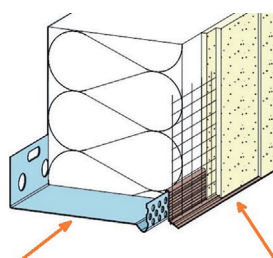
PROFILE DE DEPART ALU GOUTTE D'EAU
