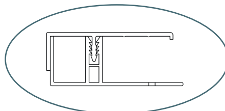
Exemple de montage ISO-EF3 + BRF
