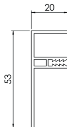
Fond commun ISO-EF3
