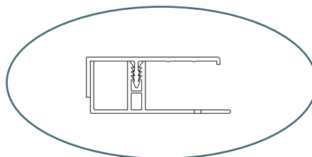
Exemple de montage ISO-EF3 + BRF3
