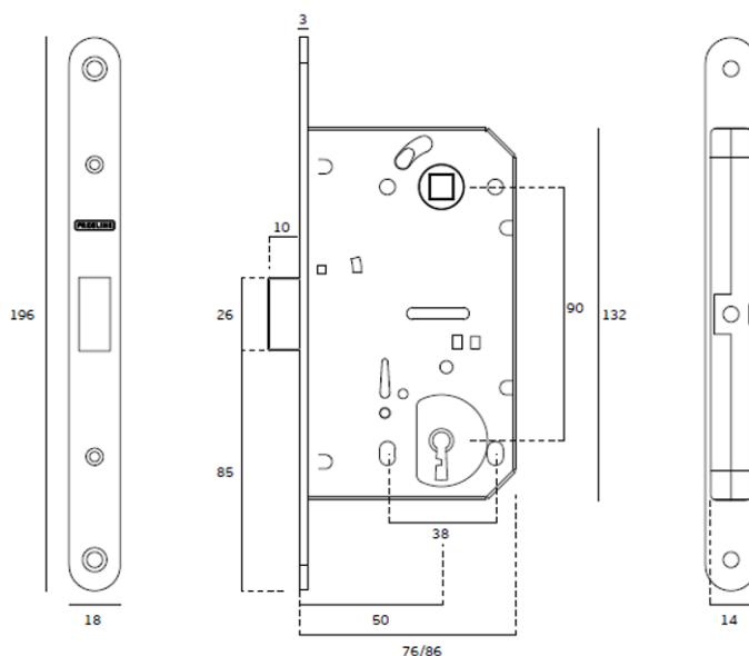
Serrure Magnétique Ref.IN.20.837.50
