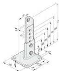
Ferrure de poteau à rotule 60/210 G
