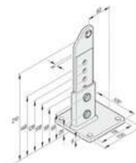
Ferrure de poteau à rotule 60/210 D
