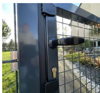
Serrure encastrée avec cylindre européen
