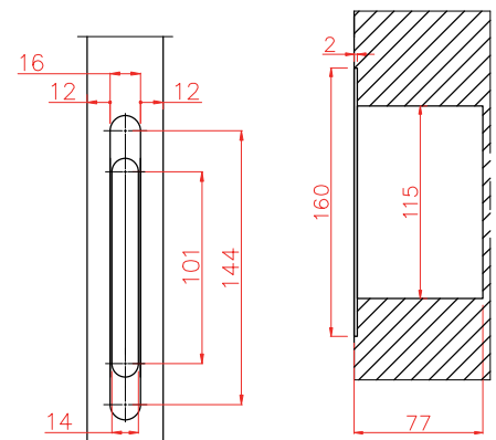
Détail mortaise
