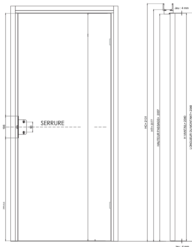
HUISSERIE MIN 50 MM
