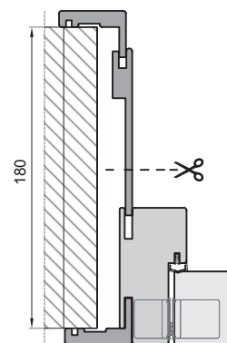
EXTENSION MAX 180 MM MAX 195 MM (2 côtés)
