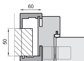
HUISSERIE MIN 50 MM
