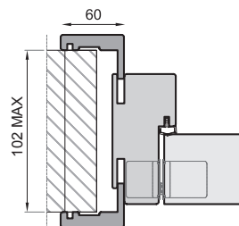
HUISSERIE MAX 102 MM
