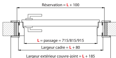
EXTENSION MAX 180 MM MAX 195 MM (2 côtés)
