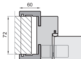
HUISSERIE MIN 72 MM
