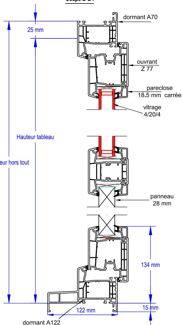
Coupe B-B :
