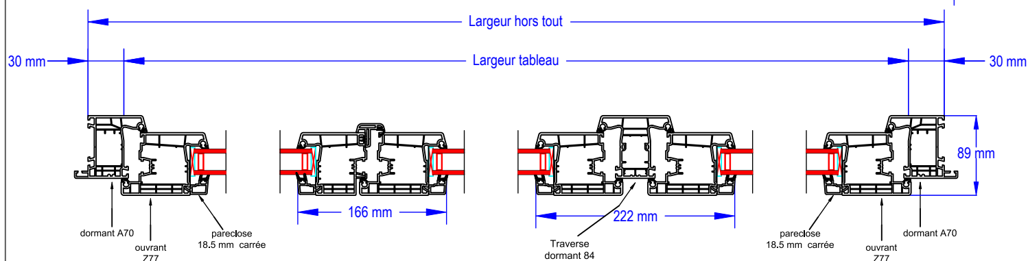
Coupe A-A :
