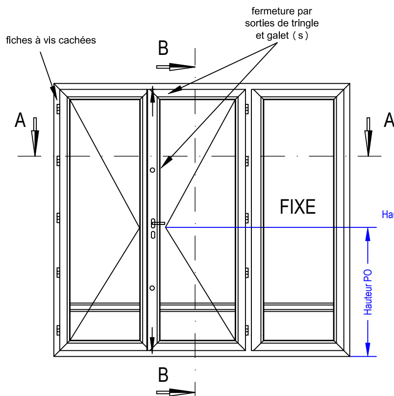
Vue intérieure :
