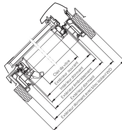
Coupe B-B
