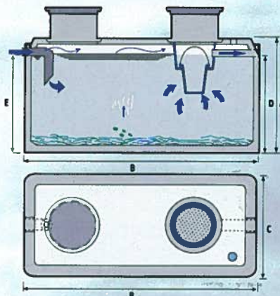
Fosse avec préfiltre incorporé et piquage ventilation
