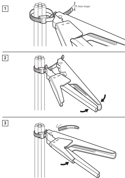
Pour serrer et couper des colliers.
