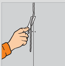
Figure 15 : Etape 5 Après séchage et expansion de la colle (12 à 36 heures) racler les bavures de colle et araser les passages de tête de vis à l'aide d'un couteau à mastic ou d'une spatule à bords arrondis.
