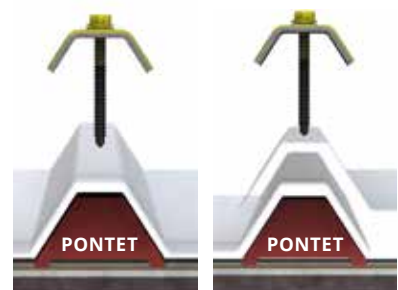
Pontet obligatoire à chaque fixation.
