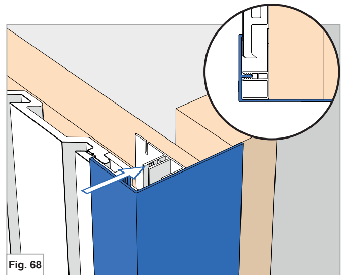
Finition d'arrêt de bardage BRC3/BRL3
