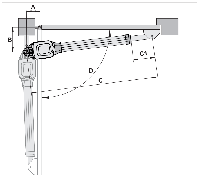
III. Dimensions en fonction des tableaux de cotes
