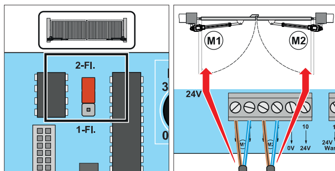
III. Deux battants
