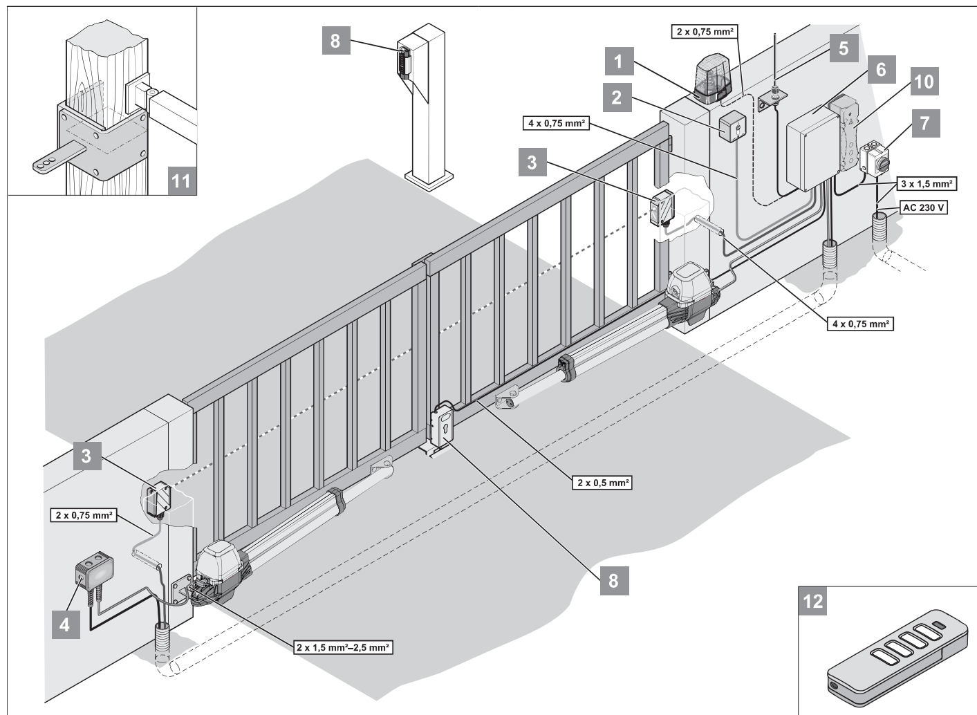
III. Structure comprenant 2 automatismes dans le cas d'un portail à deux battants
