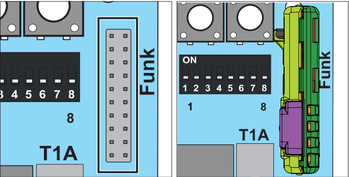
III. 1 Emplacement vide III. 2 SOMup4 S2 connecté À respecter impérativement lors du remplacement du SOMup4 S2 !
