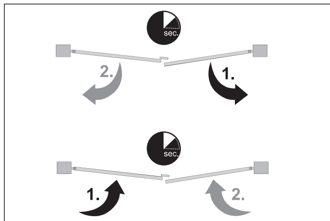
III. Exemple de séquence de mouvements
