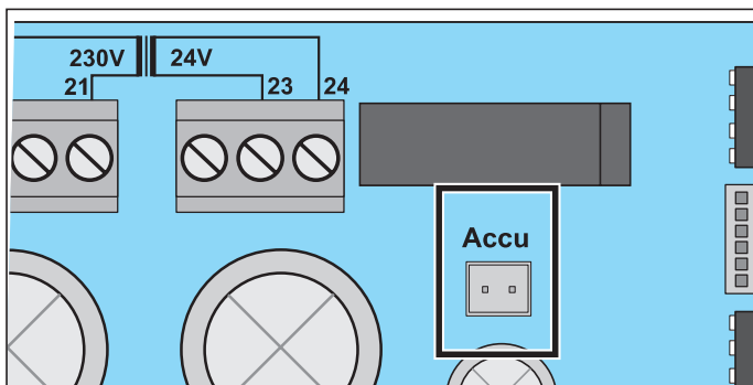
III. Raccordement pour la batterie
