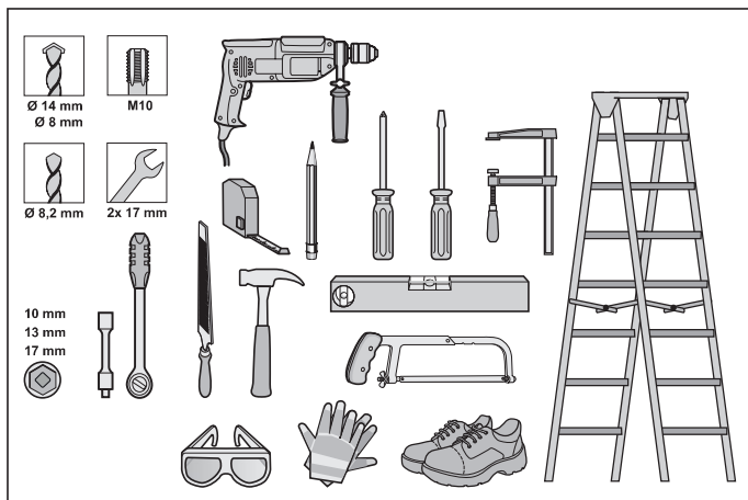
III. Outillage et équipement de protection individuelle recommandés pour le montage
