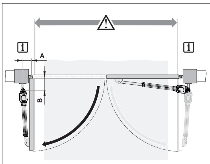
III. Ouverture de l'installation de portail vers l'intérieur
