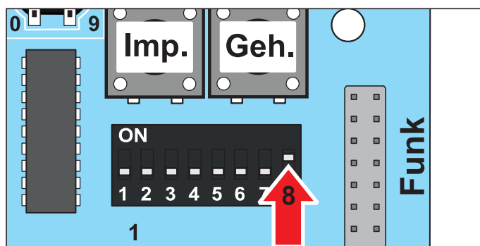
III. Interrupteur DIP 8 réglé sur "ON"
