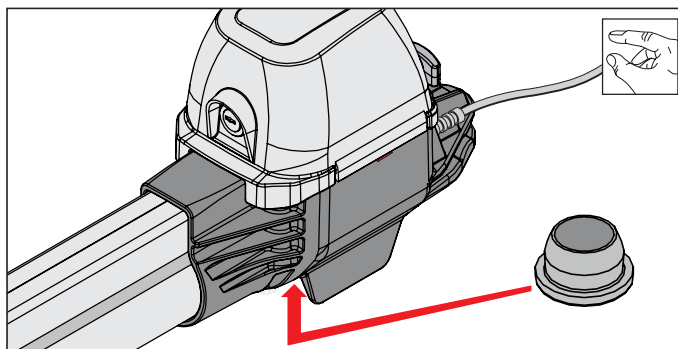
III. Bouchon – Boîtier de l'automatisme (bas)
