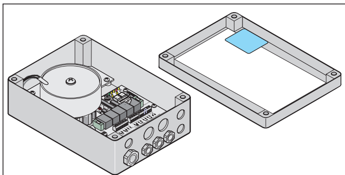
III. Commande avec plaque signalétique à l'intérieur du couvercle
