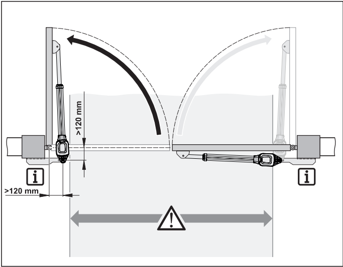
III. Ouverture de l'installation de portail vers l'extérieur
